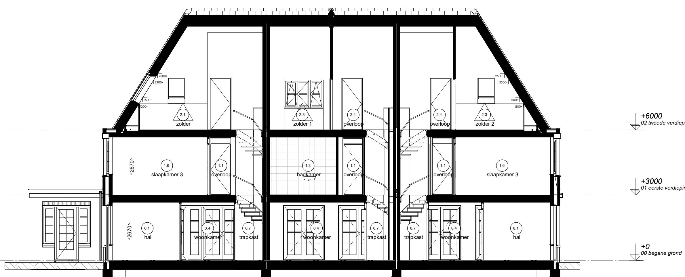
Doorsnede 17.1
