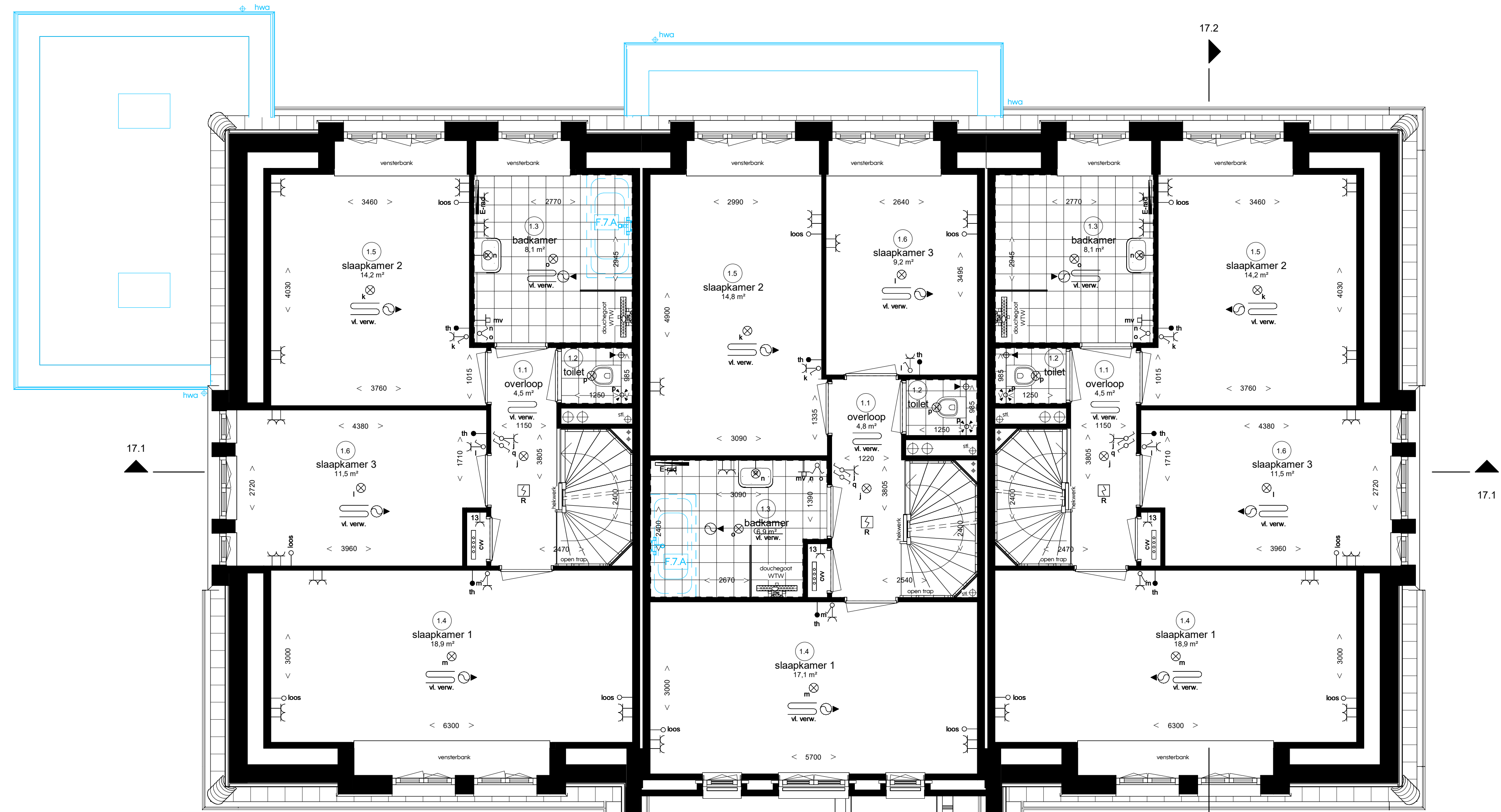
Eerste verdieping
