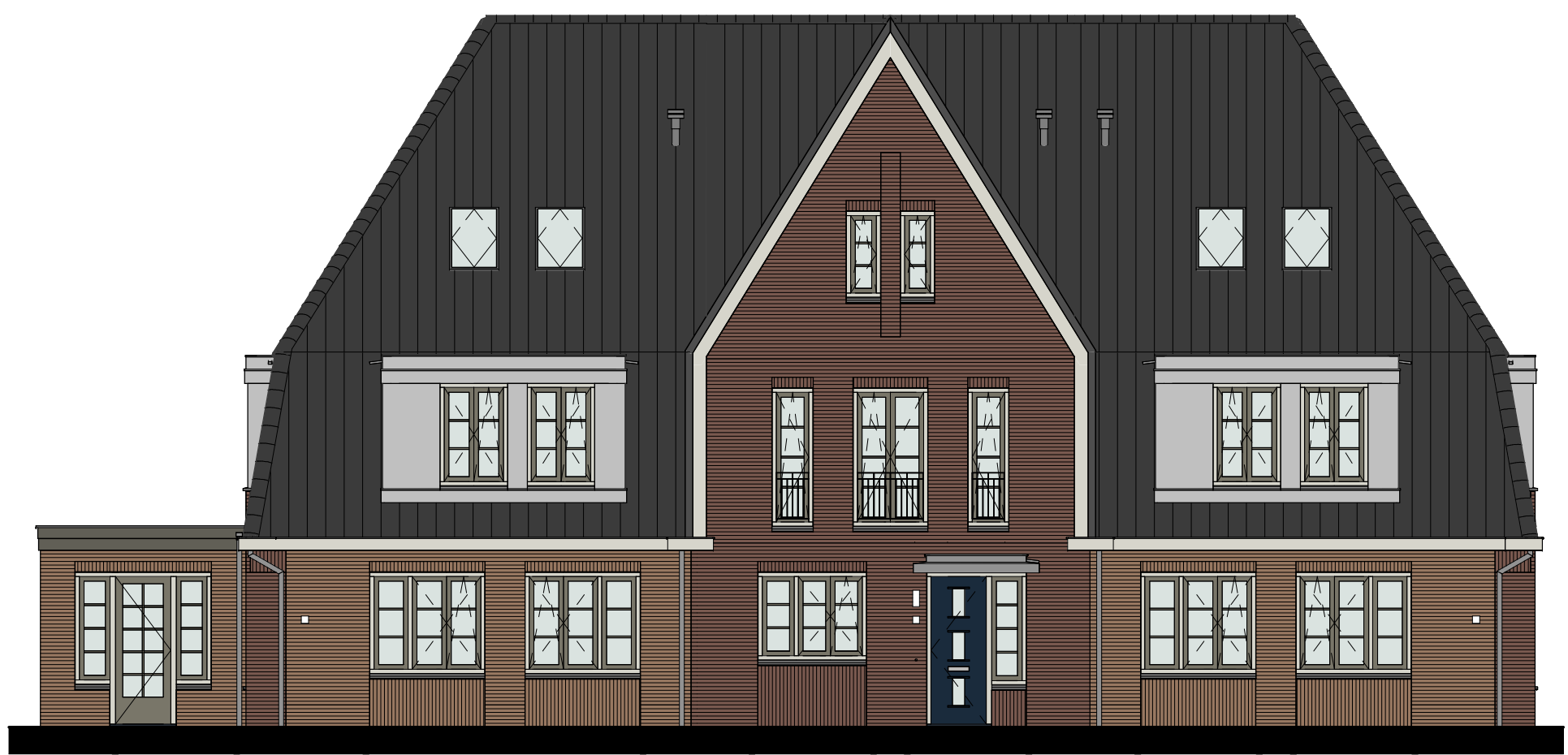
Voorgevel (Westgevel)
